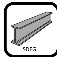
VIGA → SDFG (Sílaba Directa posición Final G)
